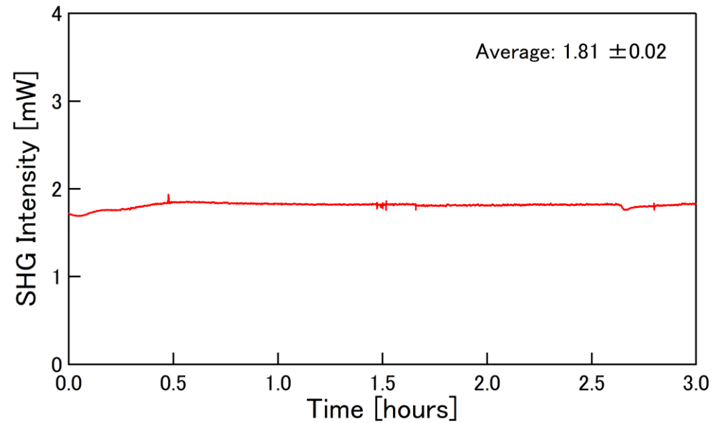
出力安定性
