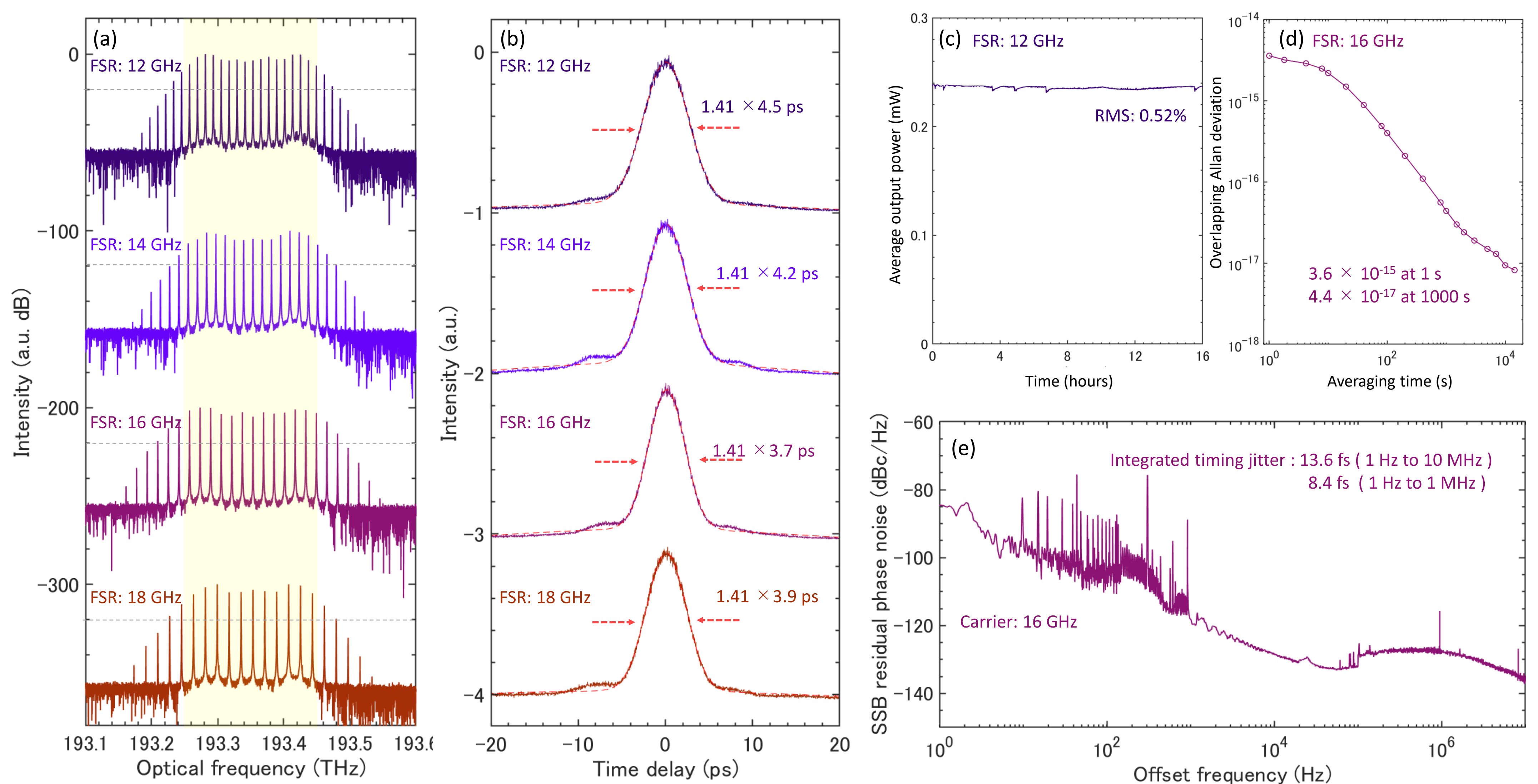
Fig. Frush の光特性の典型的な測定データ。FSR が 12, 14, 16, 18 GHz における (a) 光スペクトル（灰色点線は -20 dB ライン，黄色領域は 200 GHz 範囲），(b) パルス圧縮時の自己相関波形と該当波形をガウシアンフィッティングして得られる推定パルス幅，スペクトル波形と自己相関波形は同時に取得している。(c) FSR 12 GHz における16時間の光平均出力安定性。他の FSR でも同様の安定性を示す。平均出力安定性はスペクトル安定性と密接な関係があり，16時間における光スペクトルの変化は殆ど無いことも確認している。一般的な光学実験室環境で1時間作動後の RF 信号発生器による駆動 RF 信号波と Frush の出力光（光周波数コム）間の (d) 相対周波数安定度と (e) 相対位相雑音。
